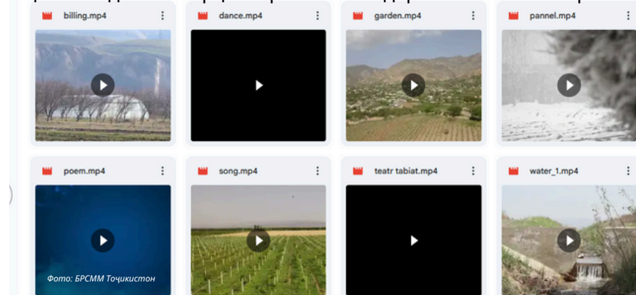
Наворҳои интерактивӣ оид ба тағйирёбии иқлим ва мутобиқшавӣ
